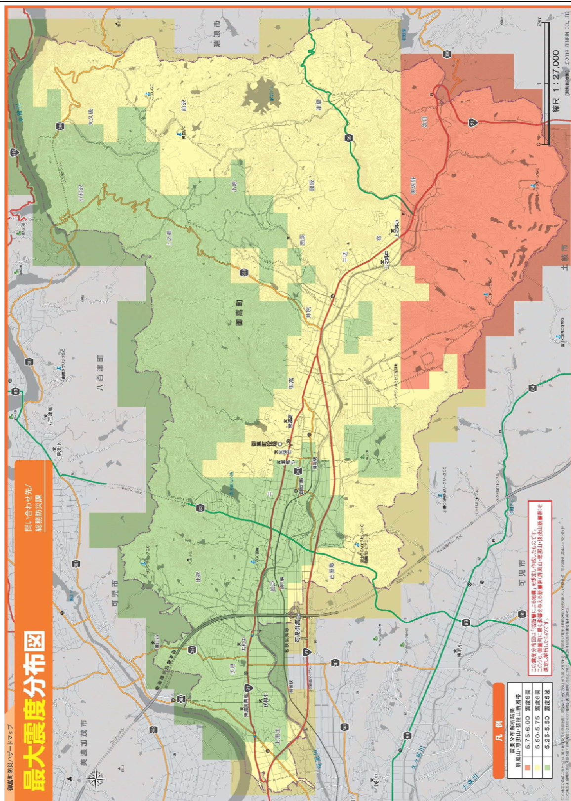
図 最大震度分布（2019（平成31）年3月作成）
