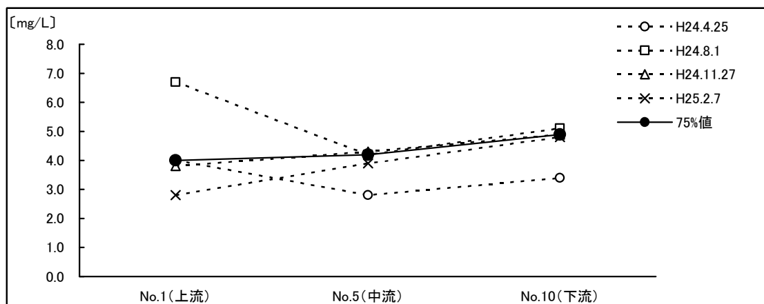
図1-9 可児川本流のCODの地点変動
