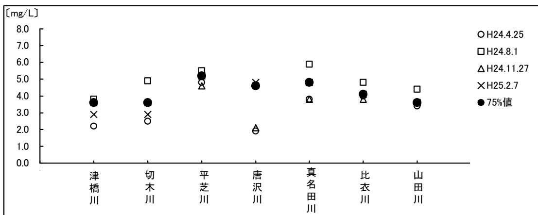
図1-10 可児川支流のCODの地点変動
