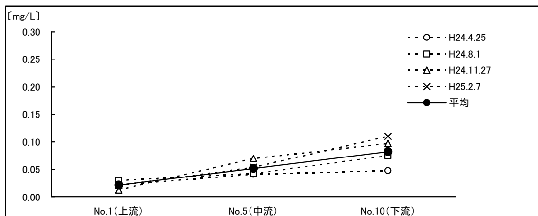
図1-15 可児川本流の全リンの地点変動
