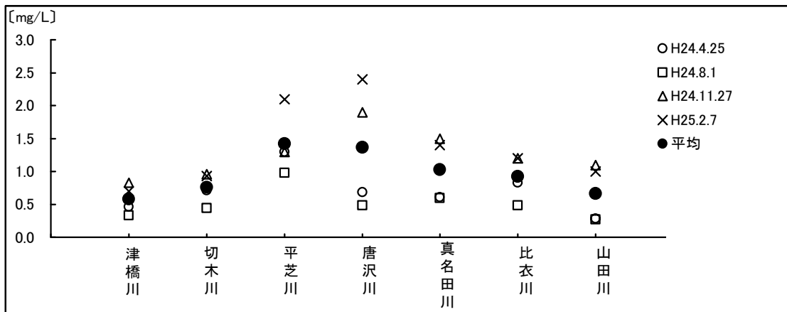
図１－１４ 可児川支流の全窒素の地点変動
