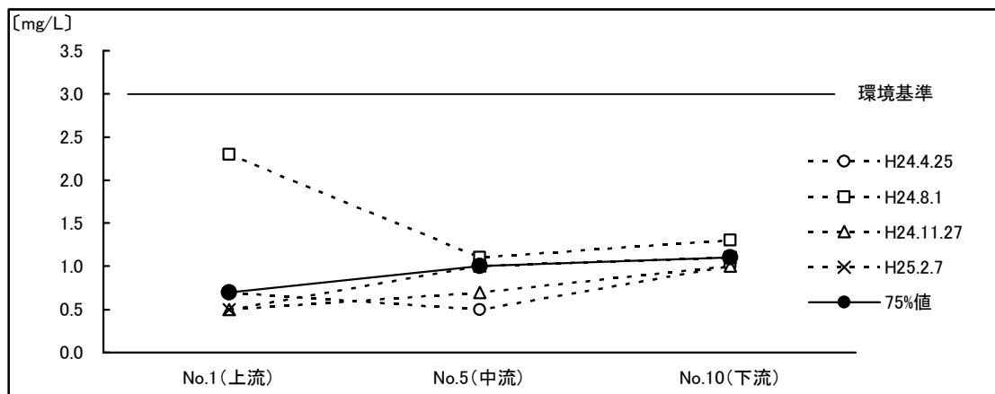
図1-7 可児川本流のBODの地点変動
