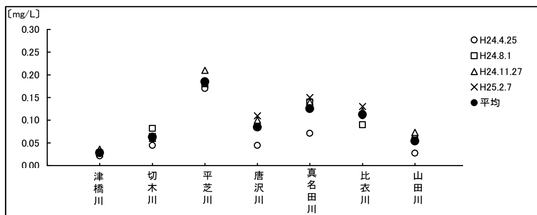
図1-16 可児川支流の全リンの地点変動
