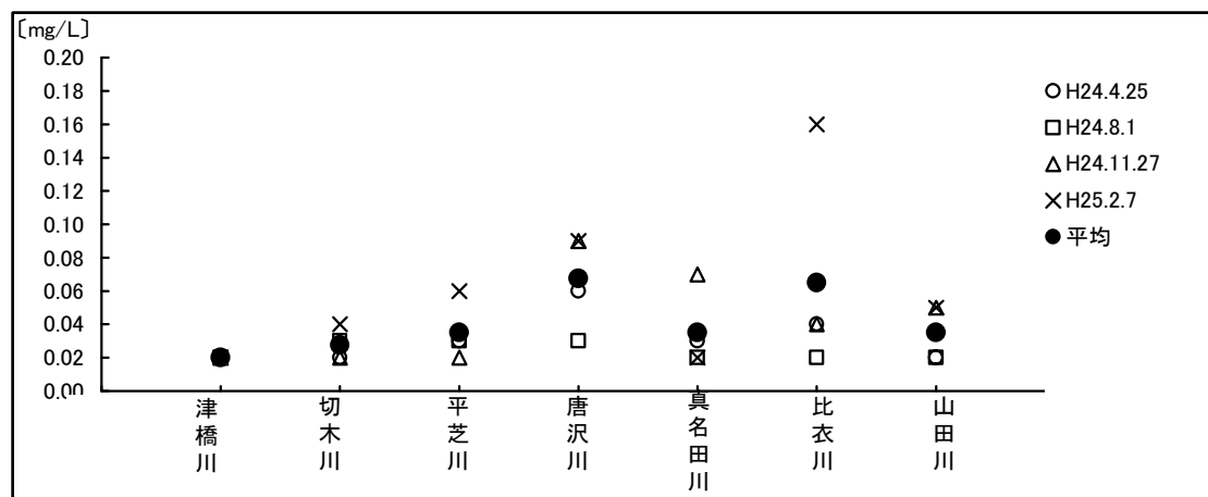
図1-20 可児川支流のABSの地点変動
