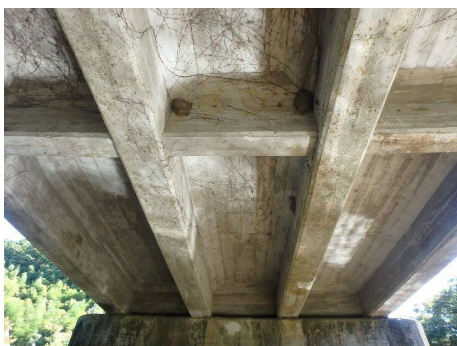
RC 橋（美佐野高橋）
