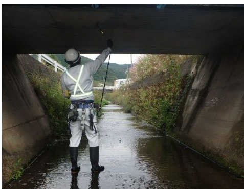
近接目視による点検状況
