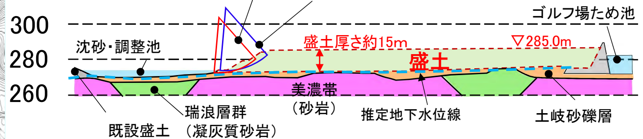
I - I' 断面
