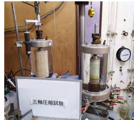
室内試験の例
