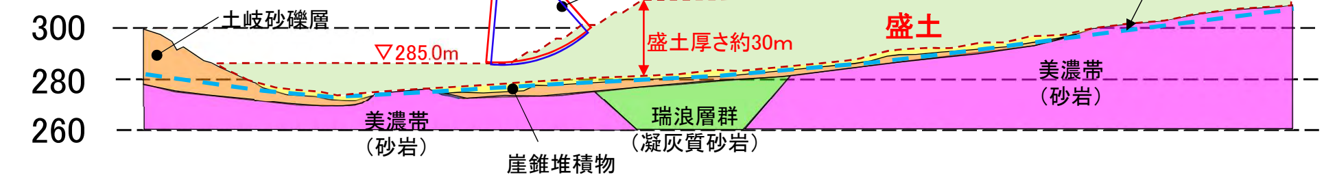
II - II' 断面
