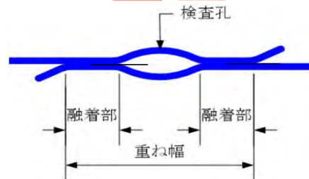
熱融着した遮水シートの接合断面例
