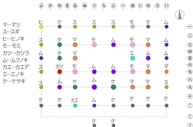
樹種鑑定結果による柱の材種
