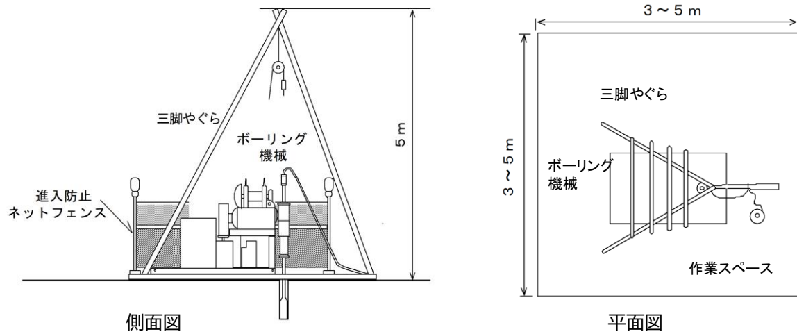
ボーリング作業状況イメージ図
